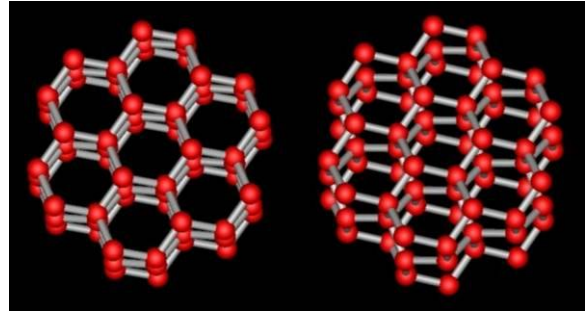
図 3 水(固相)の結晶構造図
