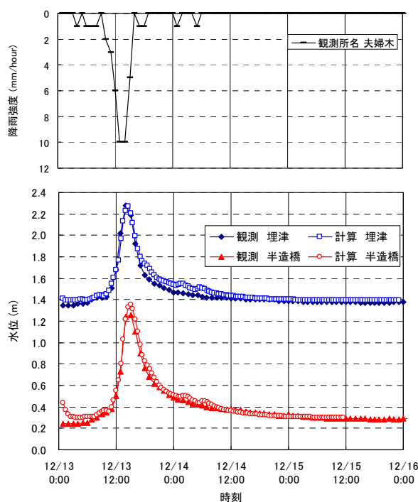
Fig. 4 ハイエトグラフと水位ハイドログラフ (計算値は数値モデルによる結果である)
