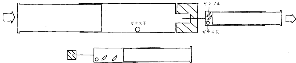
図4. 図1の注射器の針を図2の浣腸器のシリコン栓に突き刺しピストンをゆっくり引きながら還元型インジゴカーミン9 mlを移し入れ全量を10mlにする。針を上にしてピストンを押して液を少し出ししながらシリコン栓に突き刺す。これを反応管とする。
