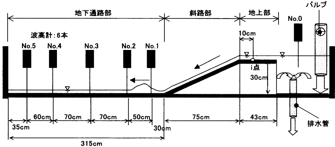
図-6 浸水実験の概要
