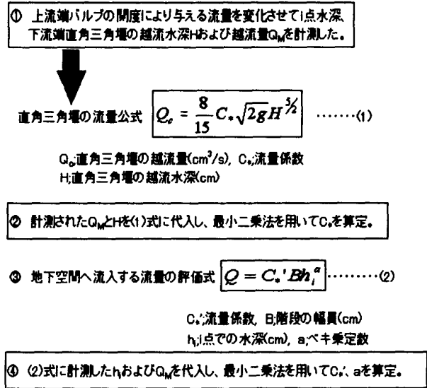
図-4 水理実験のフローチャート
