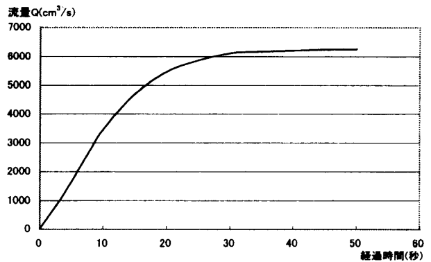
図-7 i点における流量ハイドログラフ(ケース3)
