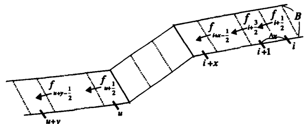
図-9 計算に用いる一次元格子
